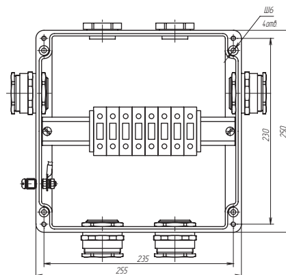
Коробка РТО 1007
