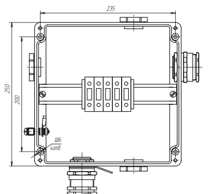
Коробка РТО 1007
